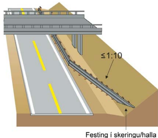
Mynd 5.4.6-1 Vegrið stagað í skeringu
